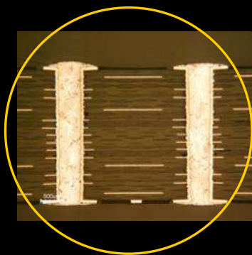
Поперечное сечение печатной платы
